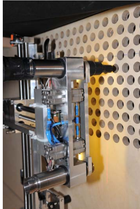
2-Achsmanipulator der Firma Delta Test
